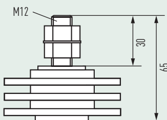
F3 - M12 x 30
