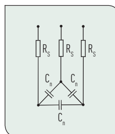
Principal circuit diagram Prinzipschaltbild
